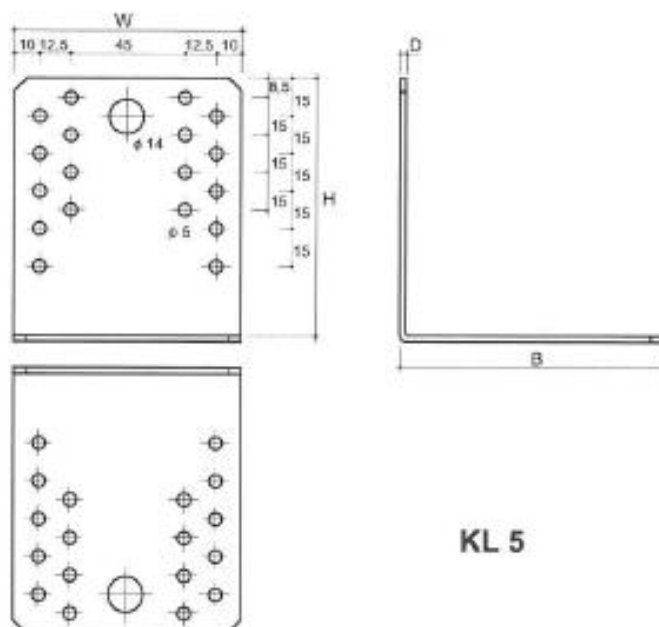
Tablica 8. Symbole i wymiary łączników DMX® typu KL
