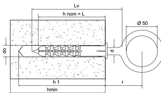
Occhiolo Ø50 - Eye Ø50
