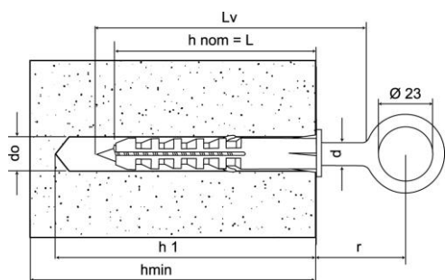
Occhiolo Ø23 - Eye Ø23
