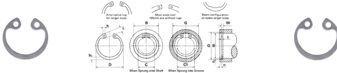
DIN 472 - D3000 Standard Internal Circlips
